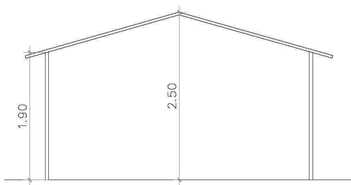
SEZIONE TIPO
